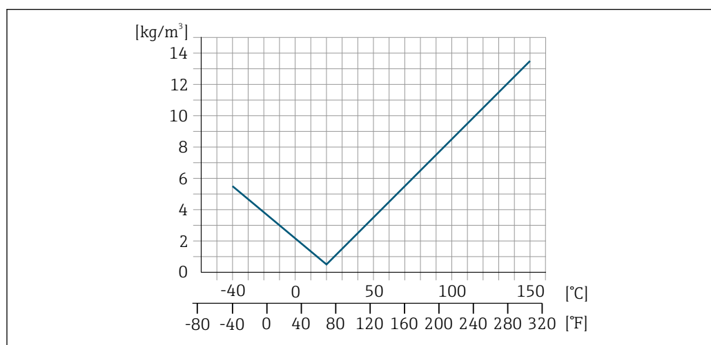
37 Калибровка по плотности на месте эксплуатации, в примере при +20 °C (+68 °F)
